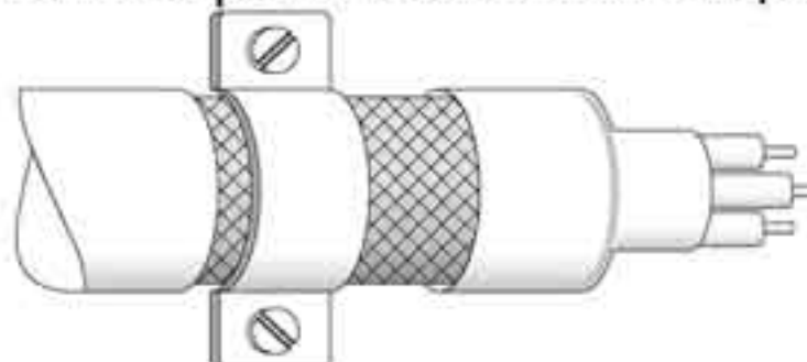
Заземление экрана на одном конце кабеля
