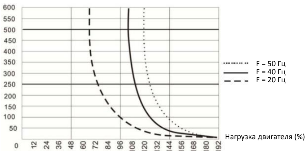
Включение защиты (с)
